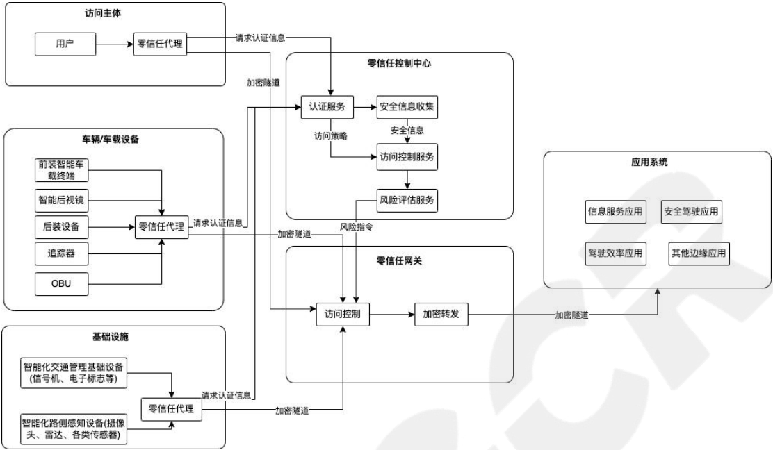
图 3 车联网零信任架构图
